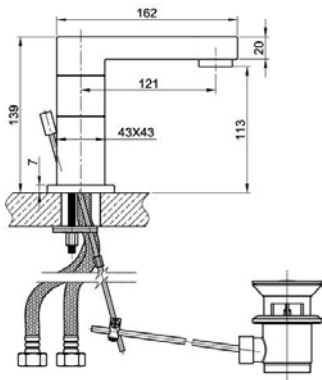
AP5001 MISCELATORE LAVABO BASIN MIXER WASCHTISCHMISCHER
