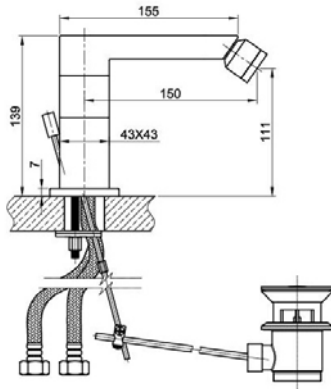
AP5002 MISCELATORE BIDET BIDET MIXER BIDETMISCHER
